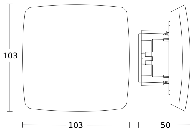
Maßzeichnung 1
